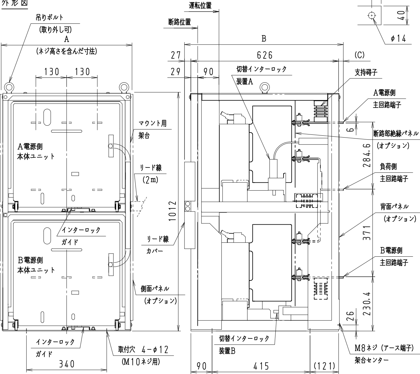
外形図
