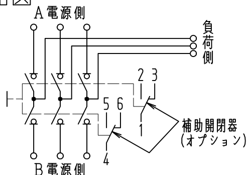
回路図
