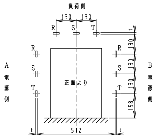
端子配列
