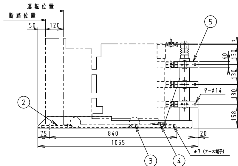
架台取付寸法及び取付ベース参考図
