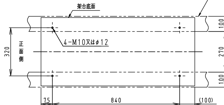
架台取付寸法及び取付ベース参考図
