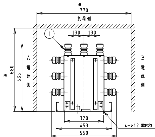
端子配列
